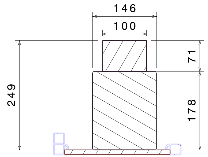
SECTION A-A Scala: 1:5
