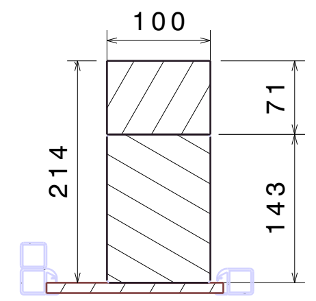
SECTION A-A Scala: 1:5
